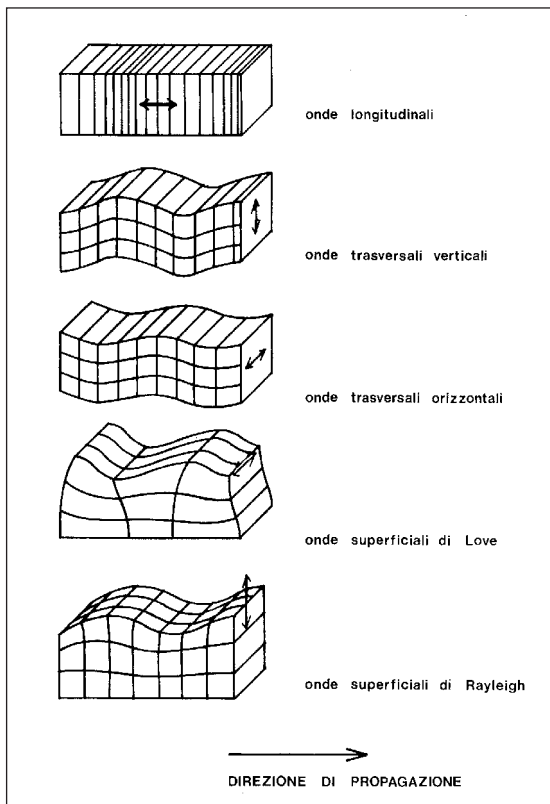
Fig. 1. Tipi di onde sismiche.
