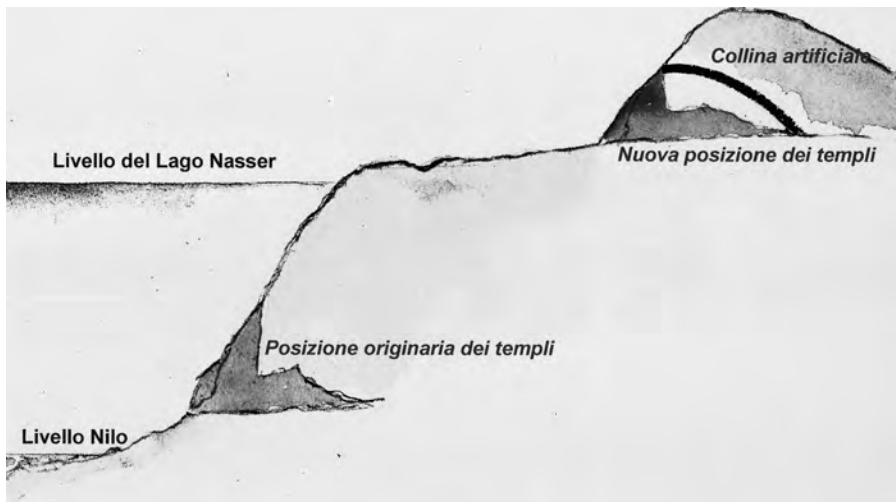
Sezione del sito di Abu Simbel con la posizione originaria e quella nuova dei templi.
